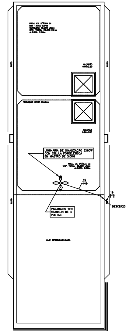
PLANTA BAIXA COB. CASA DE MAQUINAS - BLOCO C ESCALA 1:50
