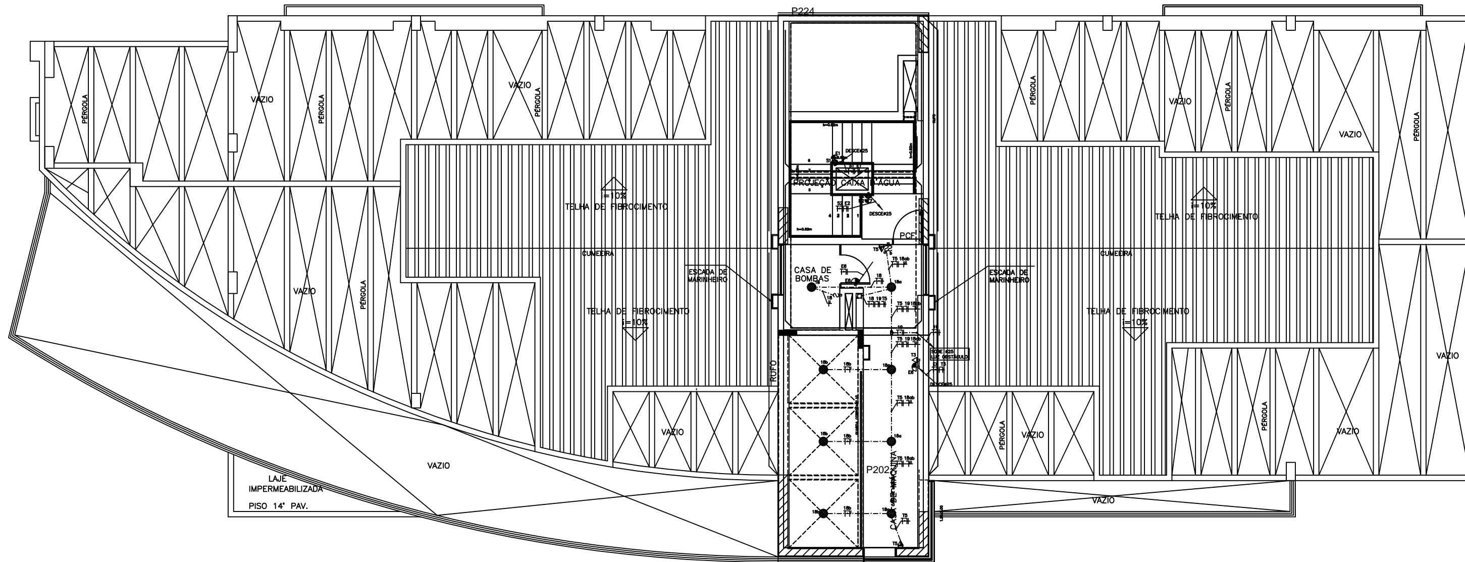
PLANTA BAIXA COBERTURA E CASA DE MAQUINAS - BLOCO C ESCALA 1:50
